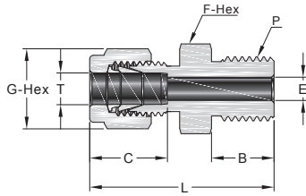
Дюймовая трубка
