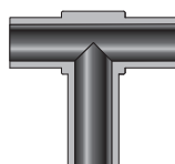
Соединительный тройник с удлиненным хвостовиком - URWU
