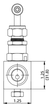
Однопортовый
